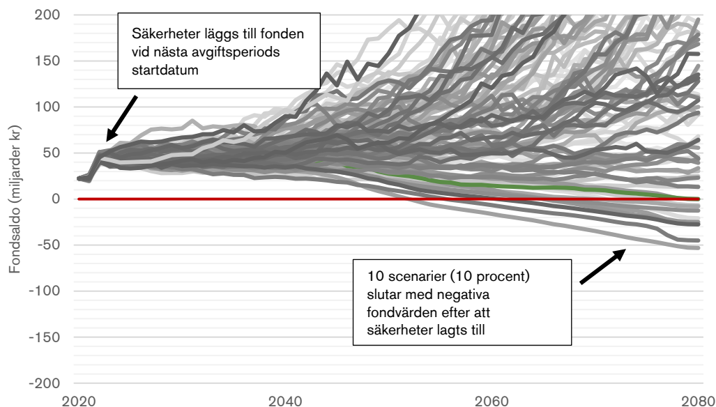
Diagram 5. Fondsaldo över tid i 100 scenarier efter att säkerheter har påkallats, där kompletteringsbeloppet beräknats med konfidensnivå 90 procent
