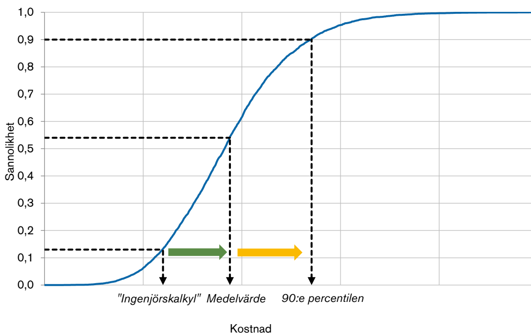
Figur 3. Osäkerhetsanalysens resultat illustrerad som en principiell kumulativ fördelningsfunktion
