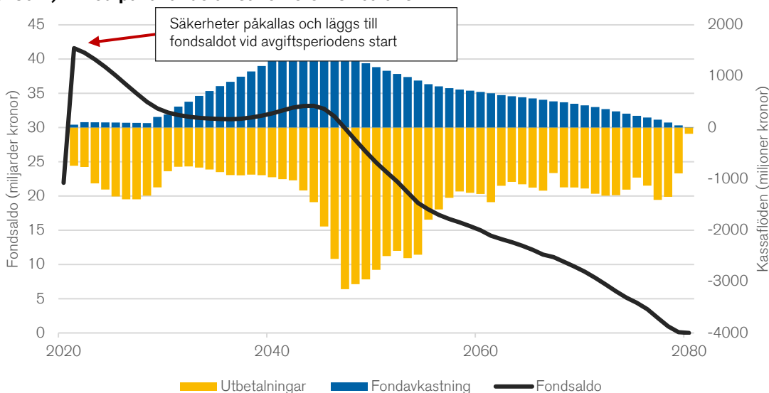
Diagram 3. Fondsaldot över tid givet att avgiftsinbetalningar upphör och utfall sämre än prognos ("chock") – med påkallande av säkerheter för balans
