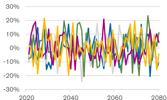
Diagram 13. Illustration av volymriskfaktor som årliga förändringstakter
