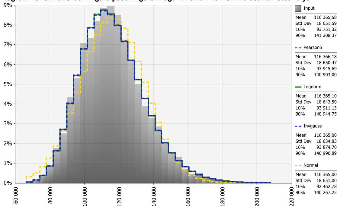
Diagram 15. Olika fördelningars passningsförmåga till utfall från SKB:s osäkerhetsanalys
