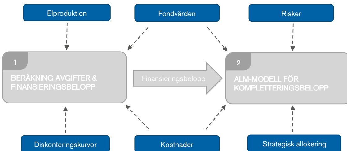
Figur 1. Beräkningssteg
